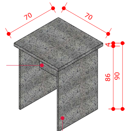
PERSPECTIVA ESCALA: 1/20
