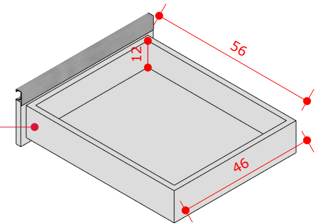
1 PERSPECTIVA - DET. GAVETAS ESCALA: 1/10
