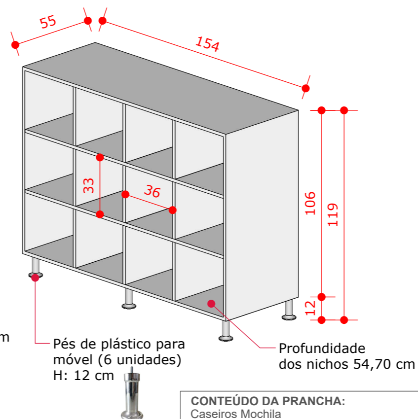
ITEM 27 PERSPECTIVA MATERNAL 2 E 3 ESCALA: 1/20 2 UNIDADES
