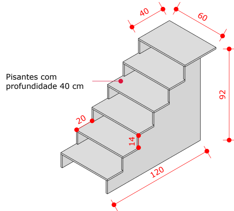
PERSPECTIVA ESCALA: 1/20
